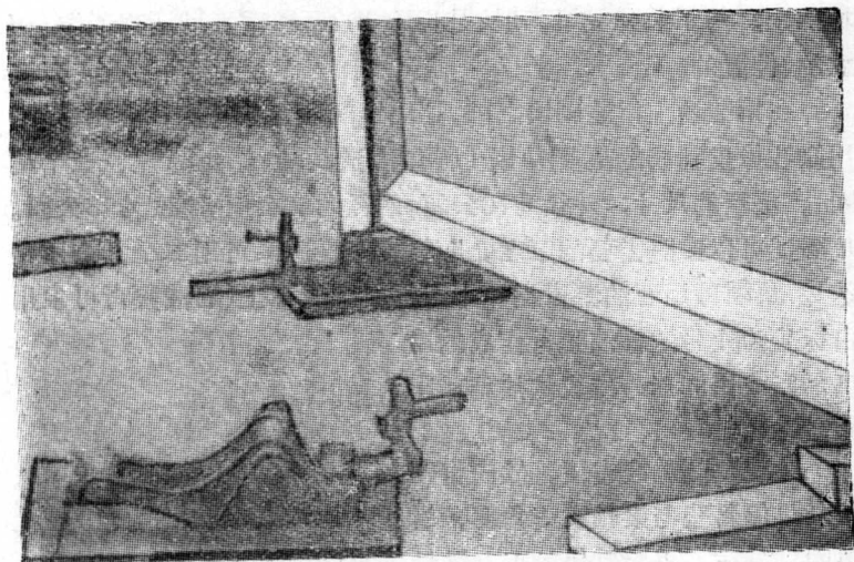
图6 在拼装场上矯正砌块用的螺旋千斤頂
