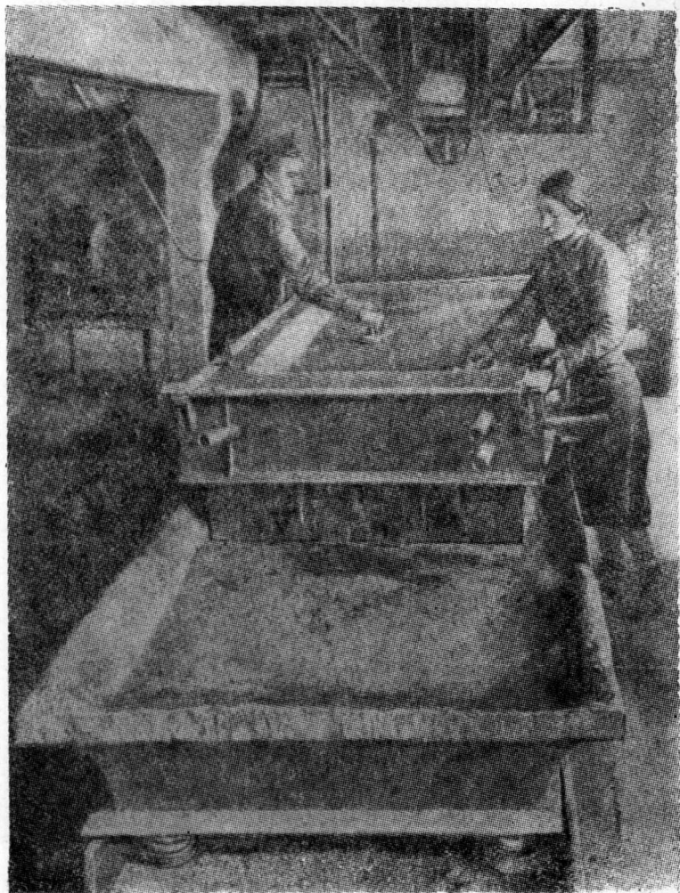
图4 梁砌块在振动台上的成型
