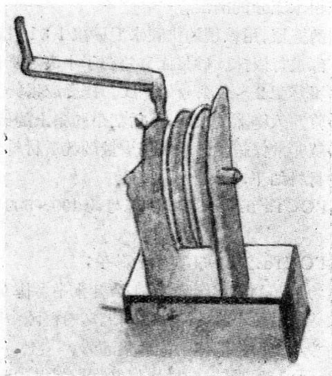
圖 8 拖拉受力鋼筋用的0.5噸手搖式卷揚機
