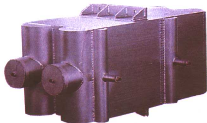
◀过冷器
