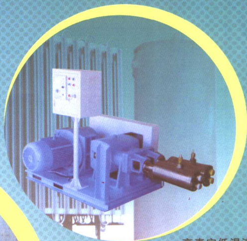
高真空低温液体泵
