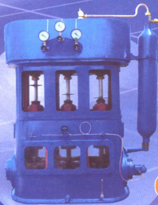
氧气压缩机
