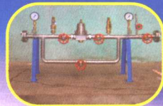
减压阀组
