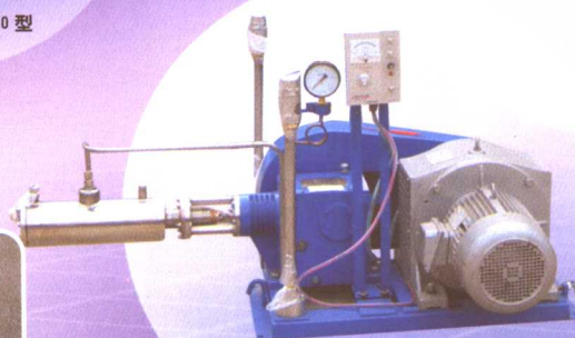
DYD80-800/165 型 低温液体泵
