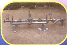
减压阀组
