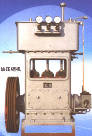
乙炔设备
