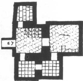
(甲) 刁家屯石室墓平面及斷面
