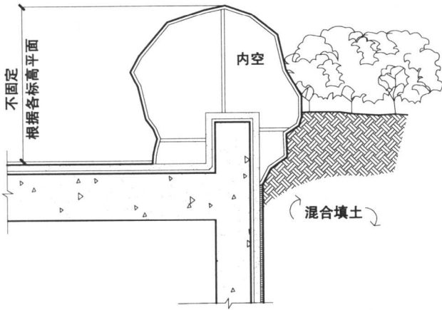
剖面图五
