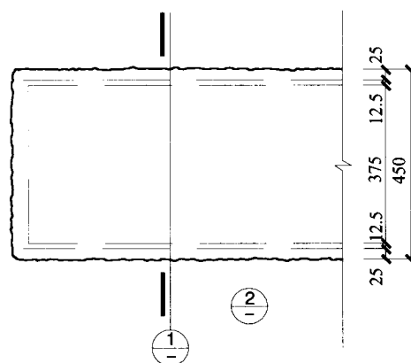
平面大样
