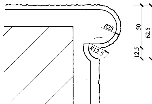
③ 大样
