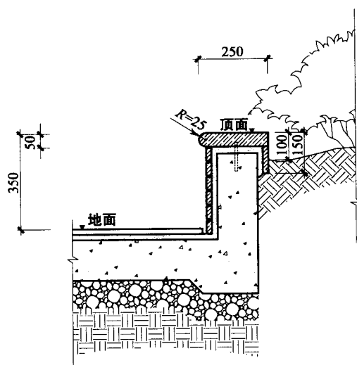
挡墙一剖面图一
