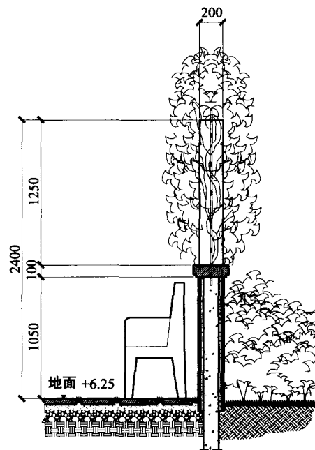
特色景观墙1-1剖面
