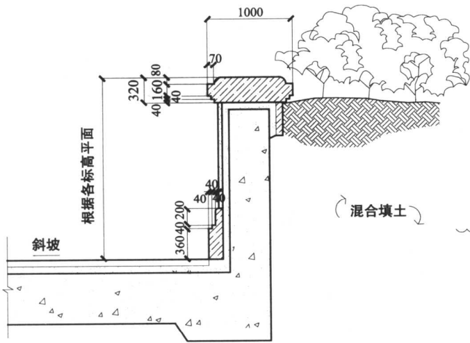
剖面图三
