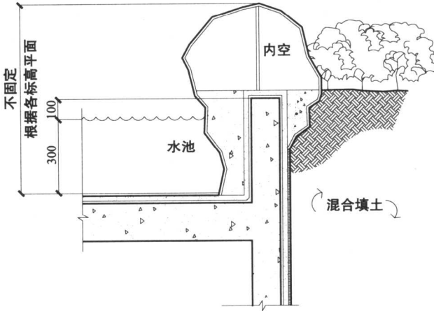
剖面图六
