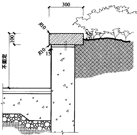
剖面图一
