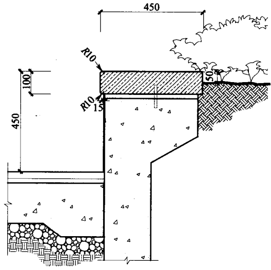
剖面图二
