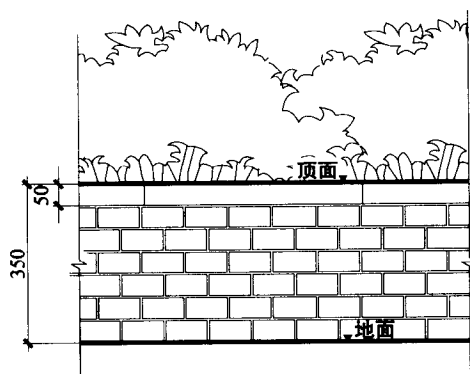
挡墙一立面图
