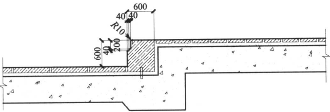
剖面图一
