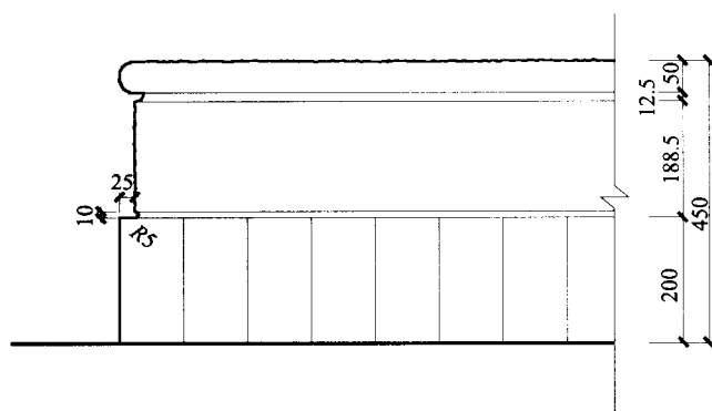
② 立面
