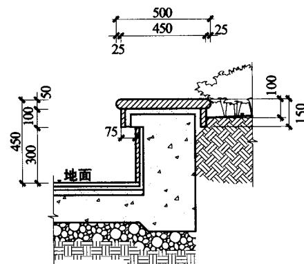
挡墙二剖面图
