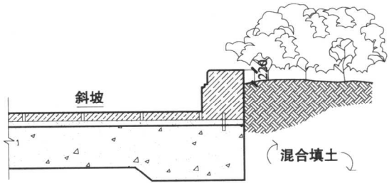
剖面图二
