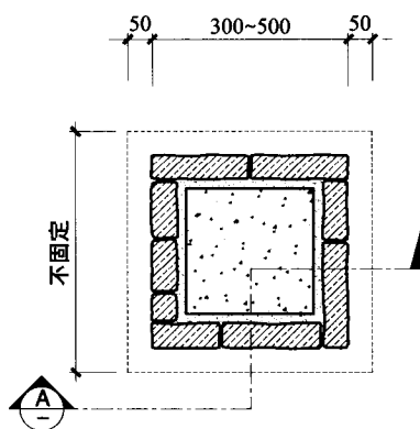
平面图
