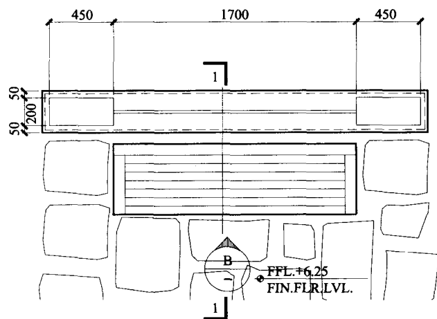
特色景观墙平面
