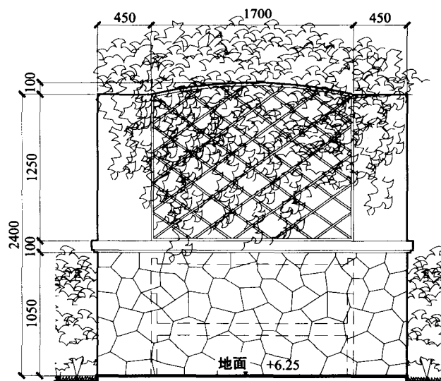
特色景观墙立面
