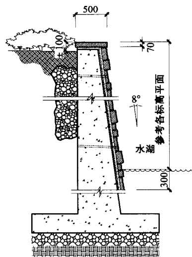
剖面图二
