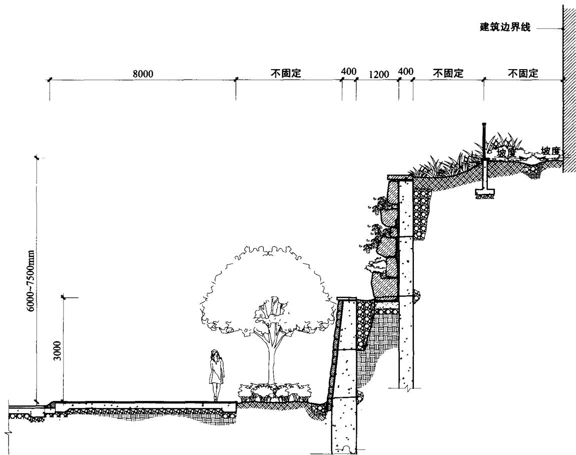
挡墙剖面图
