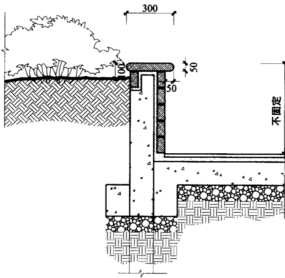
剖面图三
