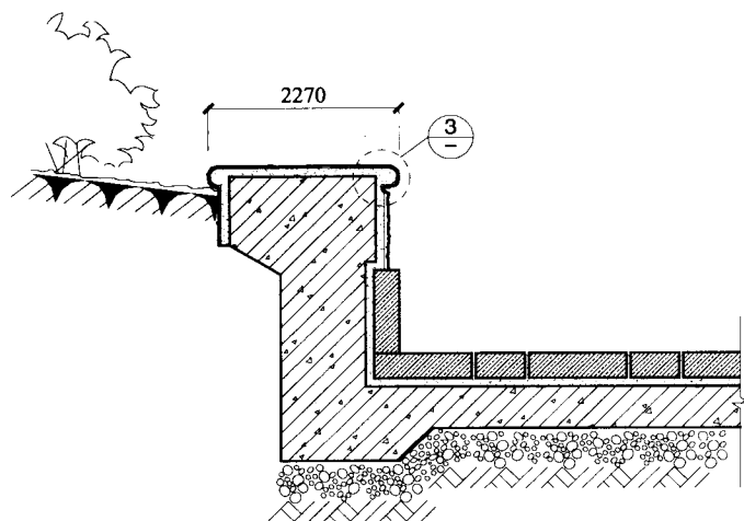
① 剖面
