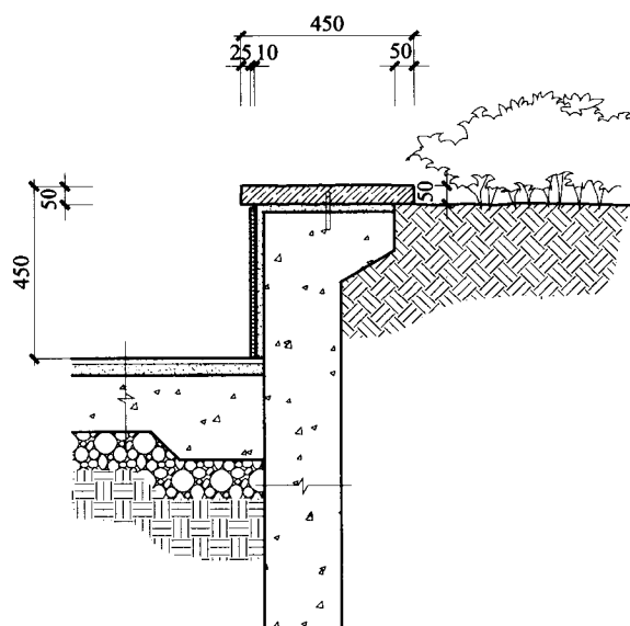
剖面图一
