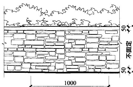
② 立面图
