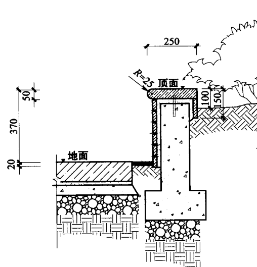
挡墙一剖面图二
