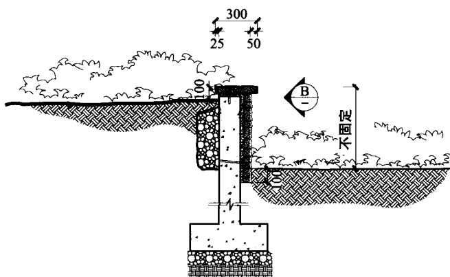
剖面图三
