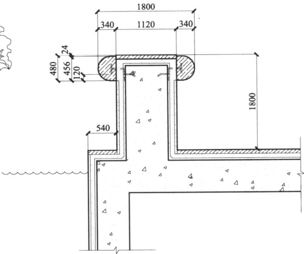
剖面图四
