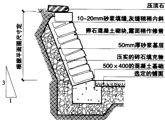
挡土墙详图
