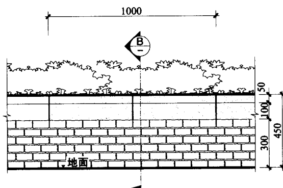
挡墙二立面图
