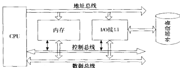
图 1-2 总线模型
