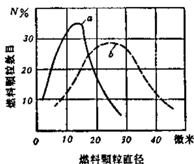
图 1-3 随喷射压力而变的雾化特性曲线 a—350公斤/厘米 2 ；b—150公斤/厘米 2 。
