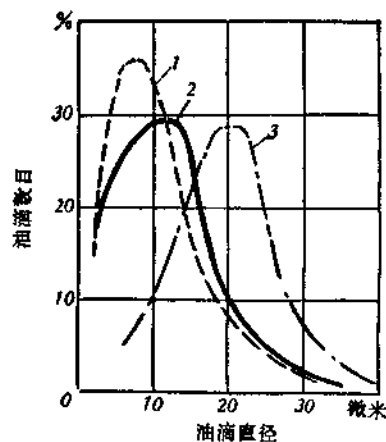
图 1—7 喷孔直径对雾化特性曲线的影响
