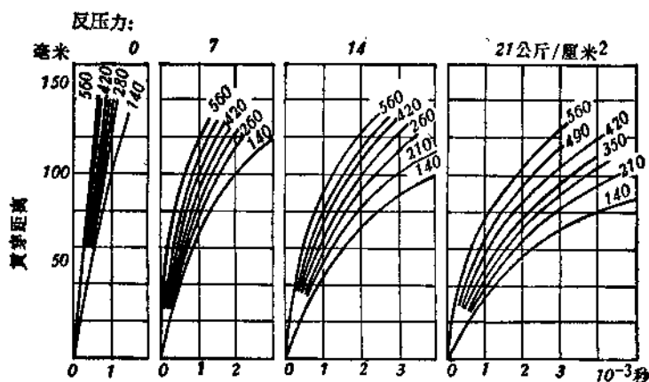
图 1-4 在不同的喷射压力和反压力下，喷注的贯穿距离随时间变化的关系
