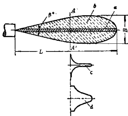
圖 1—1 噴霧焰狀體構造圖 c—沿截面 AA' 的燃料分布；d—沿截面 AA' 的速度圖。
