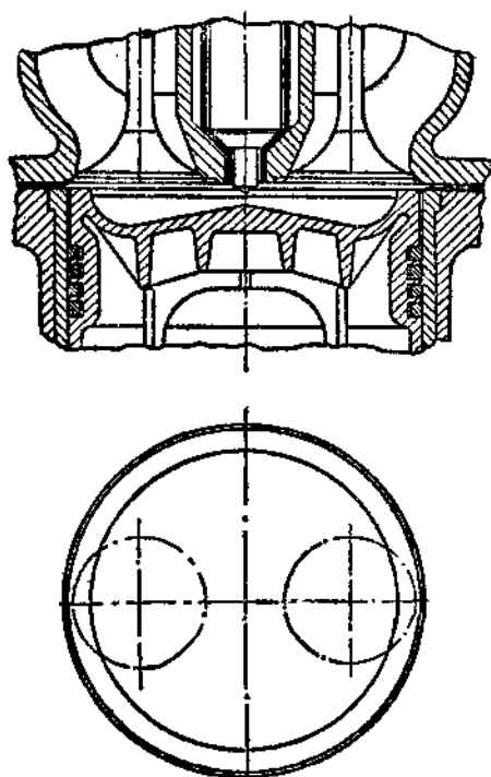
图 1-8 亚斯—204 发动机的燃烧室
