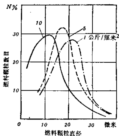
图 1—5 反压力对雾化特性曲线的影响
