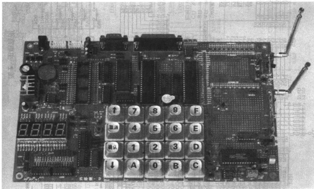
图 1 实验电路板实物照片
