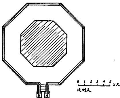
南京市栖霞山舍利塔塔座平面
