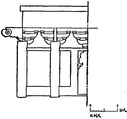
南通狼山支云塔塔壁（第五层）正立面图
