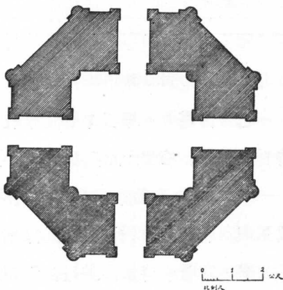
仪征县天宁寺塔底层平面
