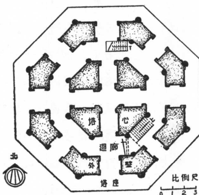
苏州虎丘云巖寺塔二层平面
