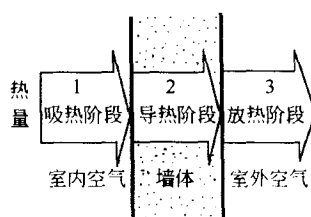
图 1-3 围护结构传热过程
