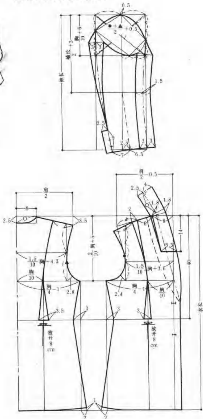
制图尺寸
