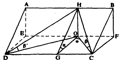
图 1-2 真倾角和视倾角的关系
