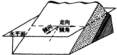
图 1-1 岩层的产状要素
