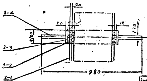
铜片安装图
