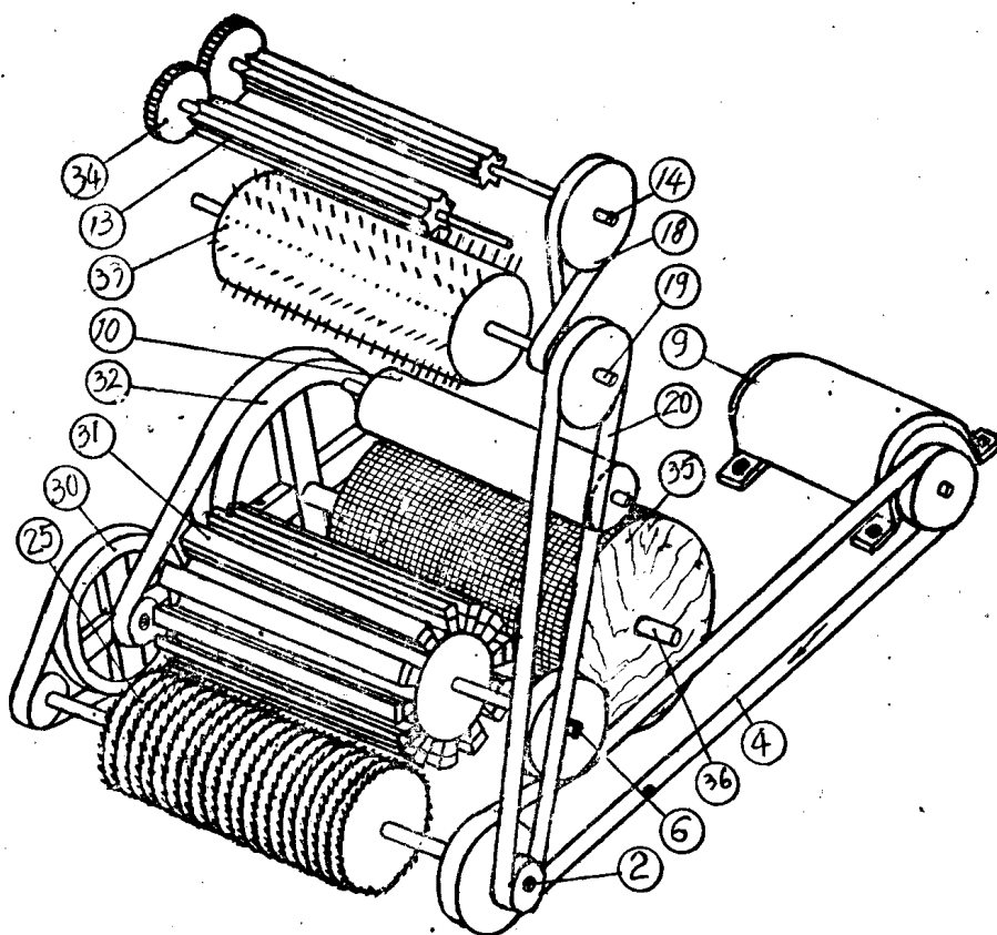
傳動示意图
