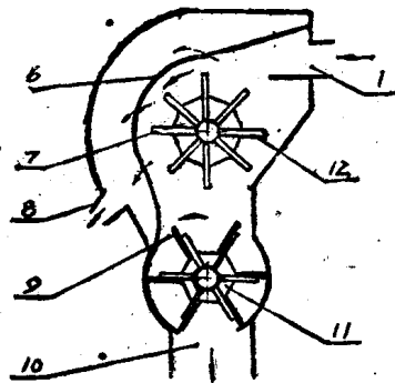
气流籽棉输送机工作示意图
