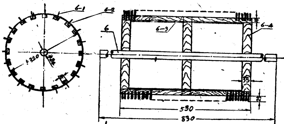
6 无刷滚筒安装图
