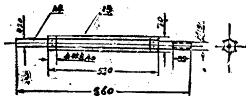
送花滚筒安装图
