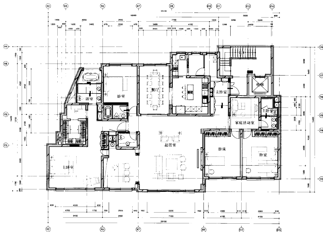
楼层平面图
