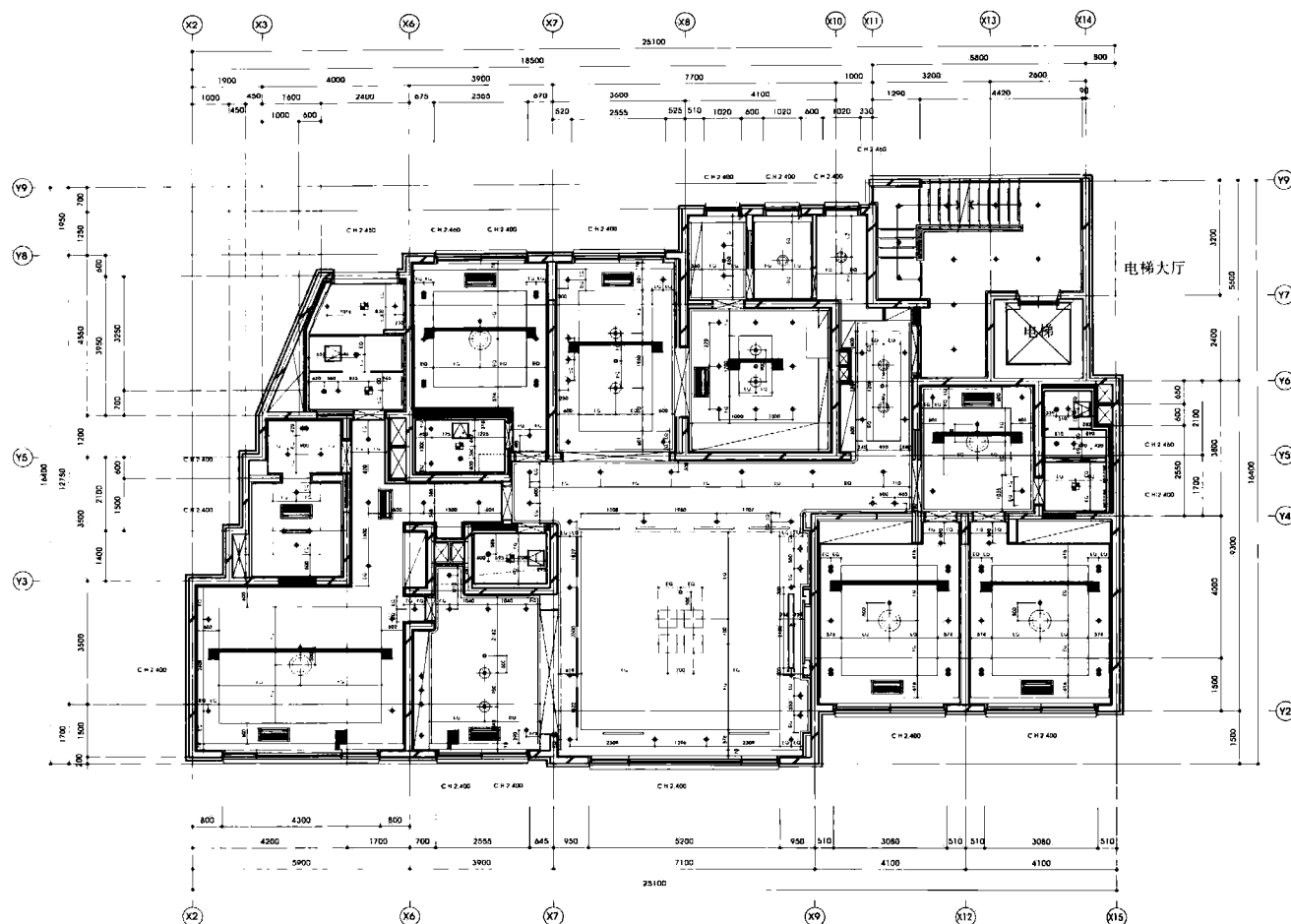
顶棚平面图
