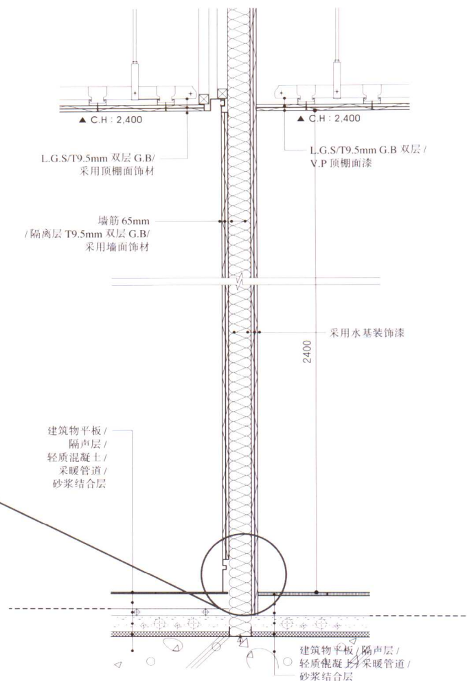
墙体剖面图(厨房和起居室)
