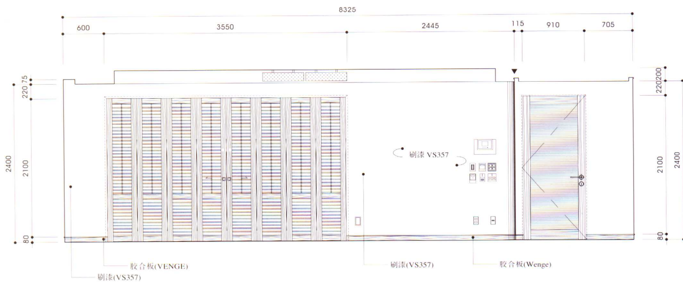
起居室立视图 4
