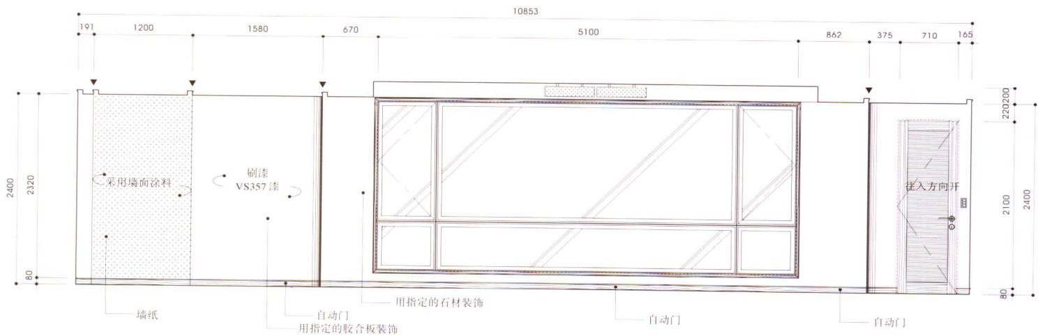
起居室立视图 1
