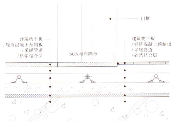
楼面板剖面图
