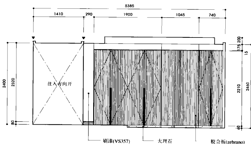
门厅立视图
