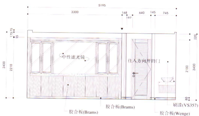
多功能厅立视图
