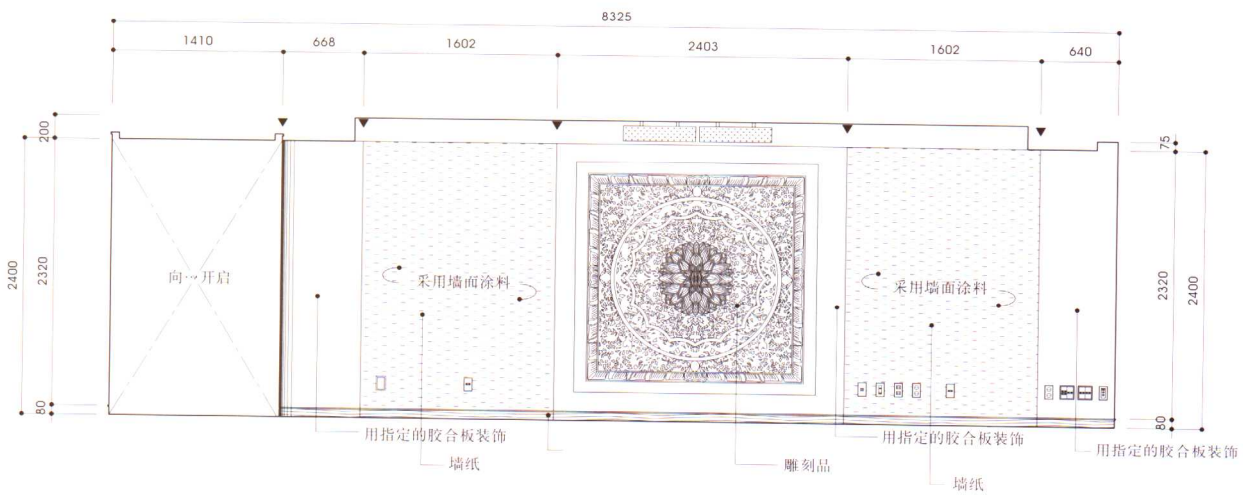
起居室立视图 2
