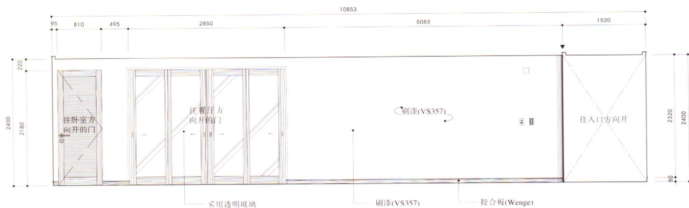
起居室立视图 3
