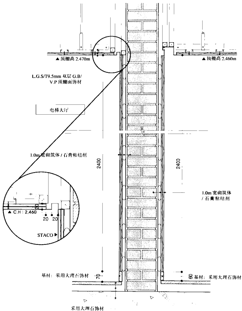
墙体剖面图(电梯大厅和入口)
