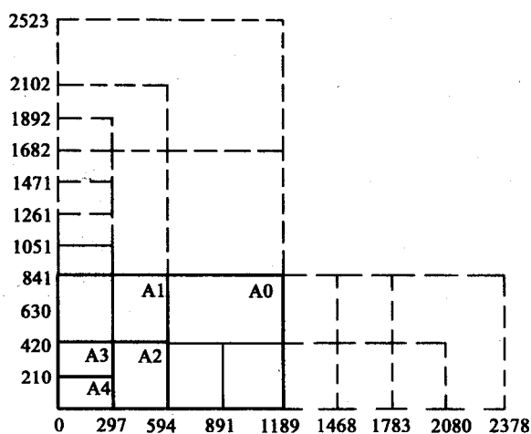
图 2-1 图纸幅面
