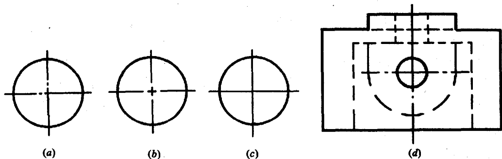
图 2-8 中心线的画法
