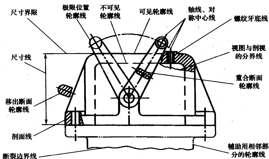
图 2-7 图线的应用举例
