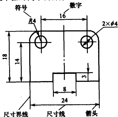
图 2-9 尺寸标注
