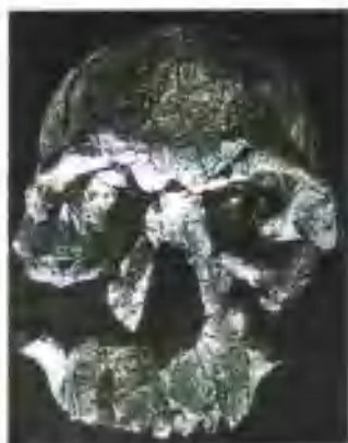
◆ 早期猿人肯尼亚人1470号人头骨化石
