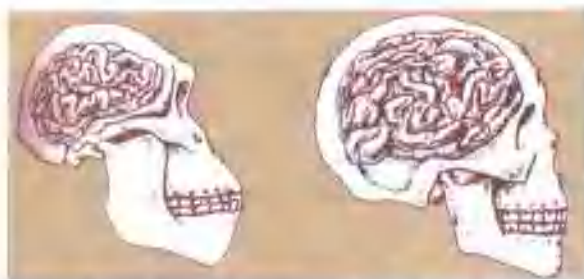
◆ 南方古猿的脑容量
