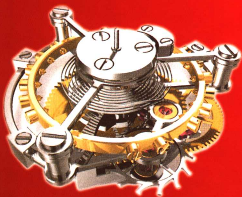
图 2-44-1 陀飞轮结构示意图
