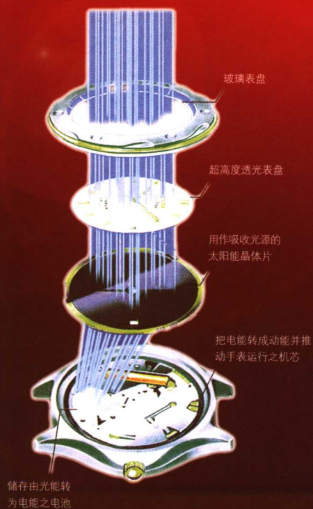
图 2-45-2 光动能指针式石英电子表
