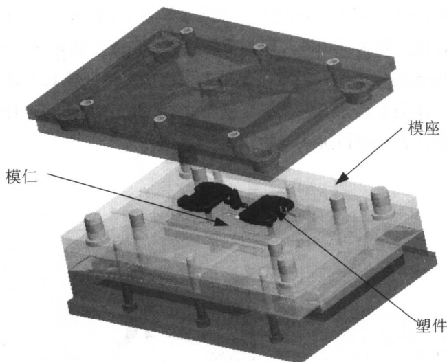
图 1.1.6 模座
