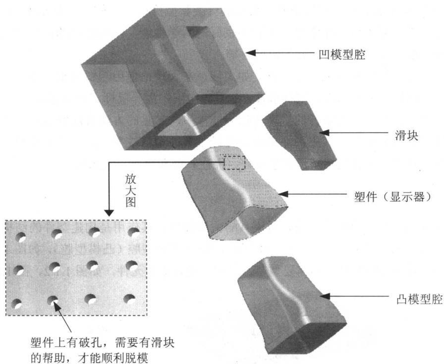
图 1.1.3 塑件成型元件 (带滑块)
