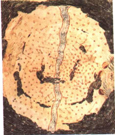
(北魏) 星象图
