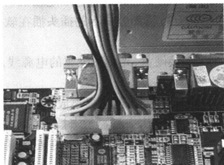
图 1-11 正确连接电源线
