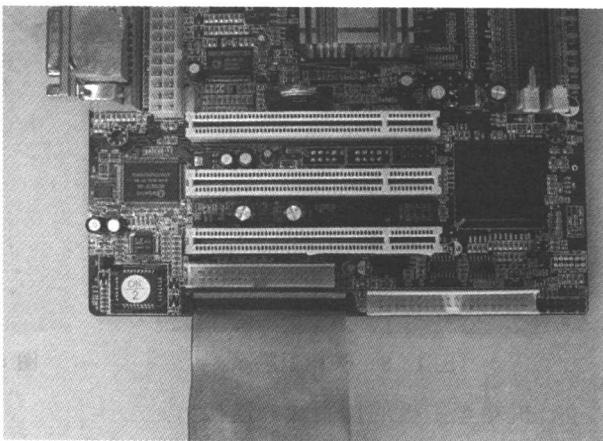
图 1-6 IDE 线的连接
