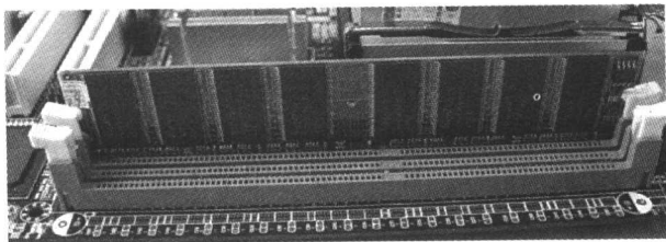
图 1-5 安装内存条
