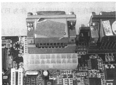
图 1-10 主板上的 ATX 电源插座
