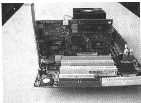
图 1-9 网卡插入主板上的 PCI 插槽
