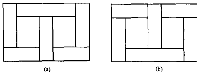
图 1-4 硅钢片
