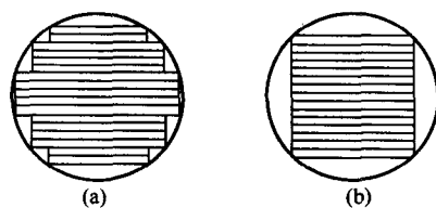
图 1-6 铁芯柱截面
