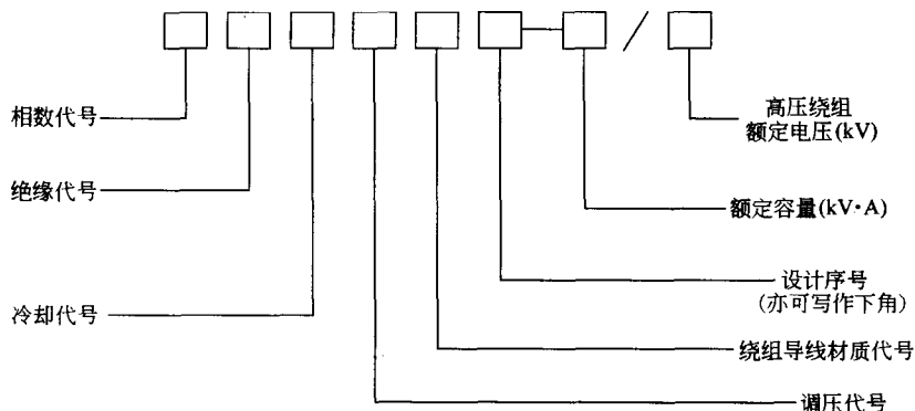
图 1-10 电力变压器全型号的表示及含义
