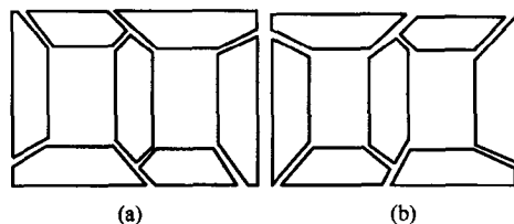
图 1-5 冷轧硅钢片的叠装法
