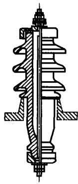
图 1-9 绝缘套管
