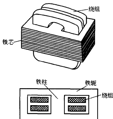
图 1-7 单相壳式变压器
