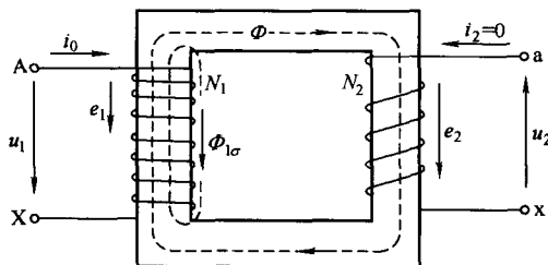
图 1-11 变压器空载运行时的示意
