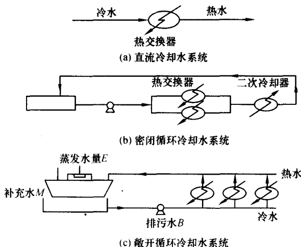
图 1-1 不同类型的冷却水系统示意图
