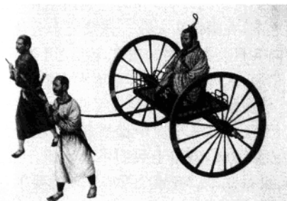
春秋时期木犂车复原图
