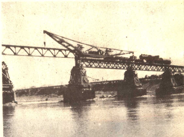
蘭(州)新(疆)鐵路的黃河便橋正在積極修建中。
