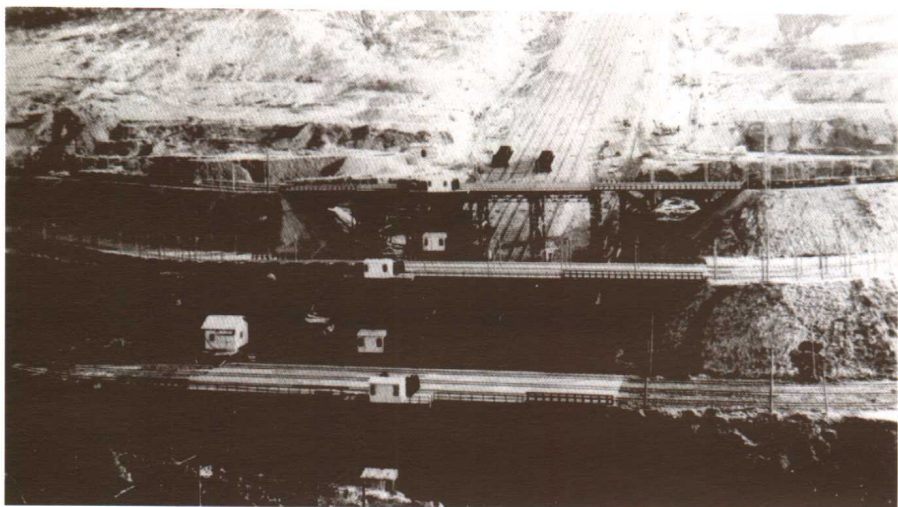
抚顺煤矿露天采煤提升系统,惯称为东、西大卷。三道平行电铁路的下面是大煤仓。各掌子生产的煤炭运来此处,翻入煤仓,然后运至地面。摄于1931年10月19日。
