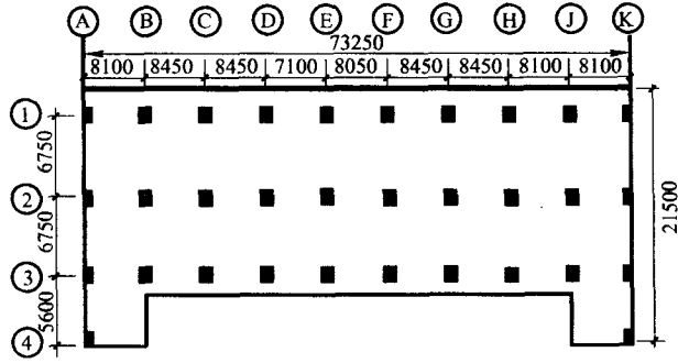
图 1-9 Harbour Cay 板柱建筑平面示意
