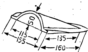
犁鏵另件圖
