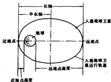
人造地球卫星运行轨道示意图
