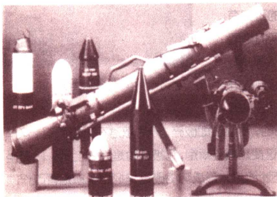
瑞典 81 毫米无坐力炮
