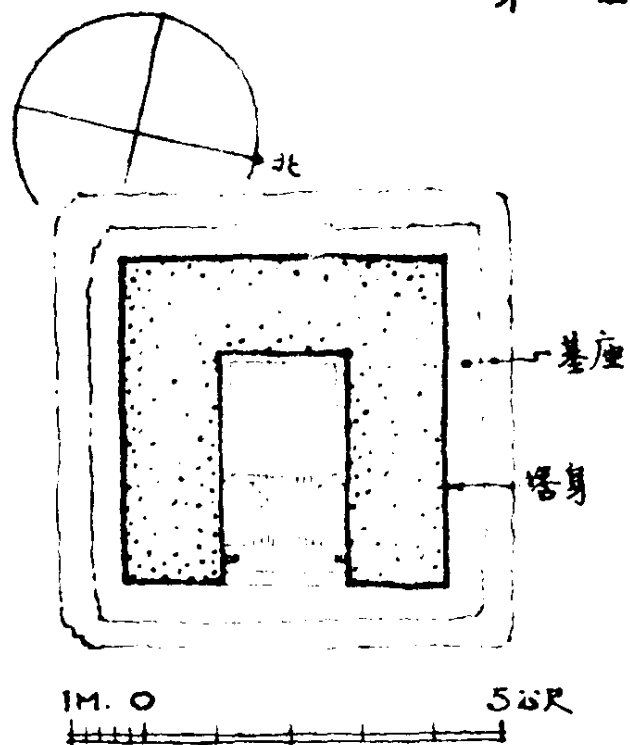
雲南大理縣佛面寺塔平面。
