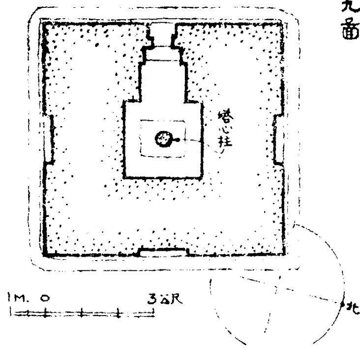
雲南大理宏聖寺塔平面圖。
