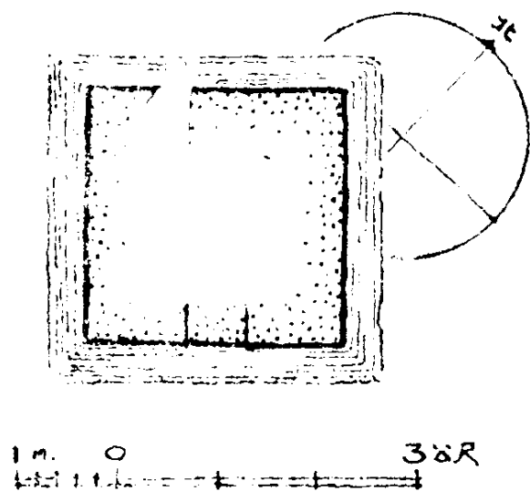
雲南昆明市妙應蘭若塔 平面圖
