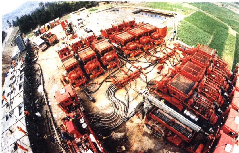
酸化压裂施工现场
