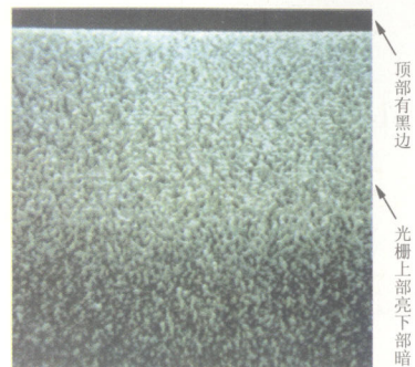
图38 场升压不足
