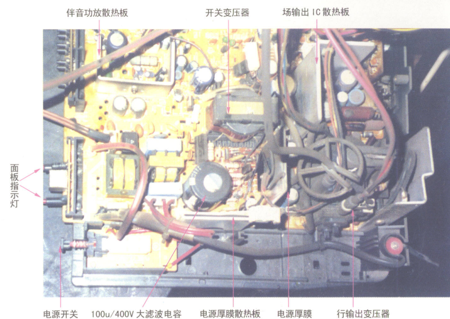
图50(a) 整机底板实物图
