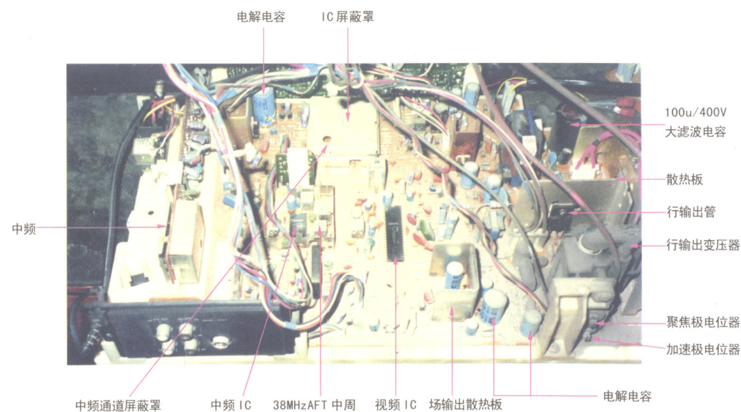
图50(b) 整机底板实物图
