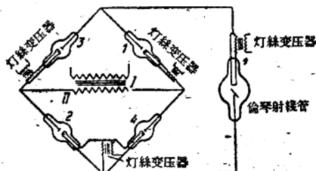
图 3. 4K-110-00 型倫琴射綫設備的高压电路原理图。
