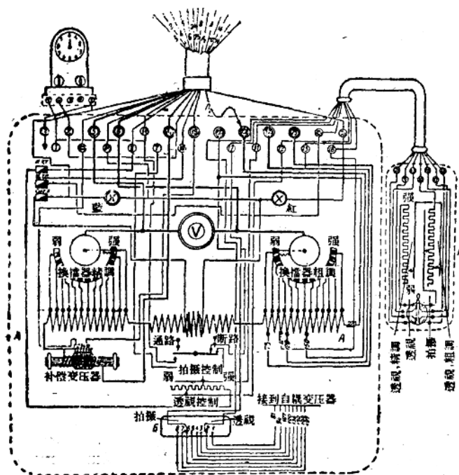
图 2. 4K-110-CO 型倫琴射綫设备的配电台电路图。
