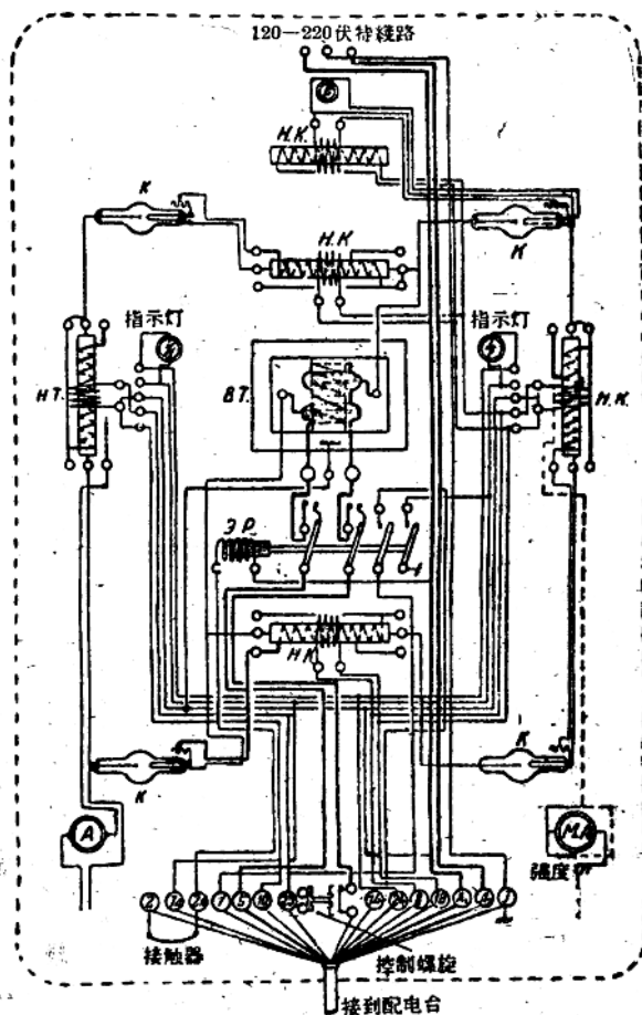
图 1. 4K-110-00 型倫琴射綫设备的电路图。
