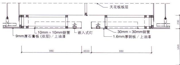
1层天花板照明—剖面图B及立面图
