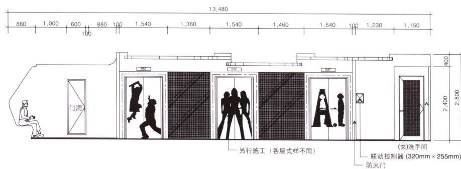
立面图
