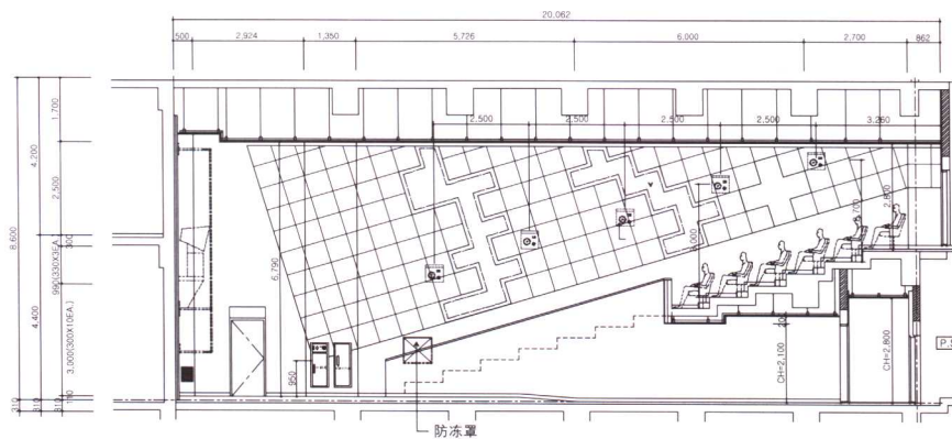
立面图
