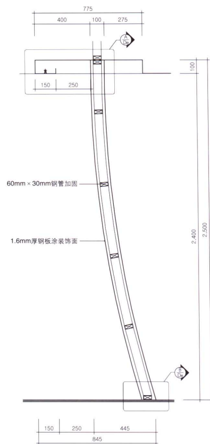
剖面图A
