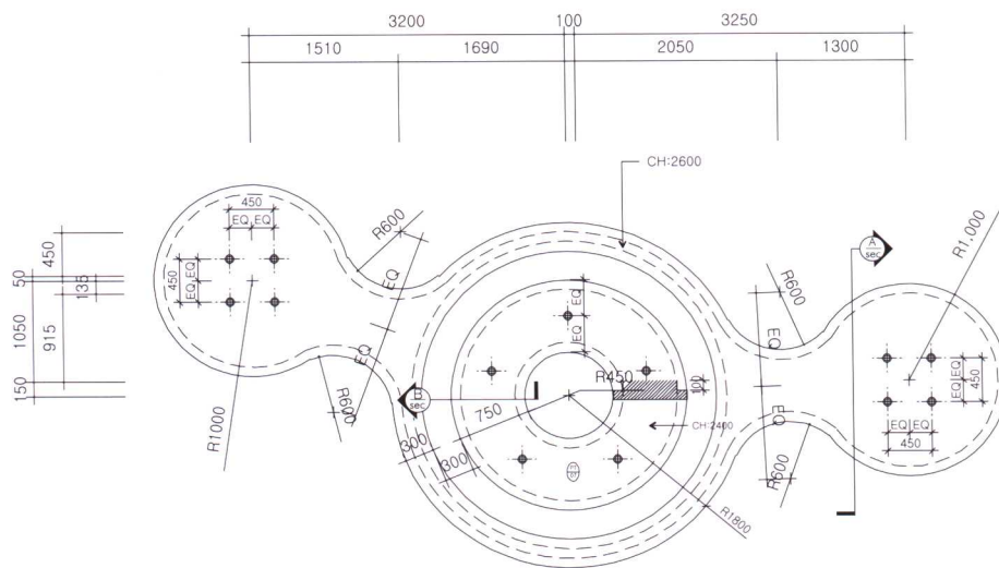
天花板局部一平面图
