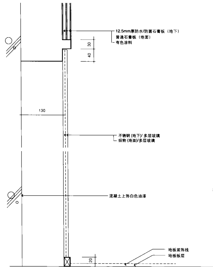
墙体—大样图
