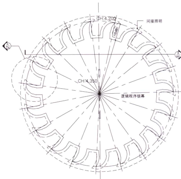
1层天花板照明—大样图A及主视图
