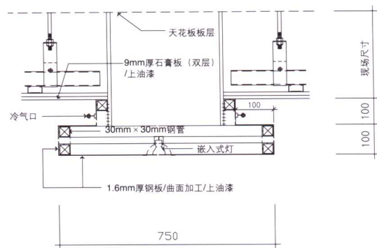
剖面图B
