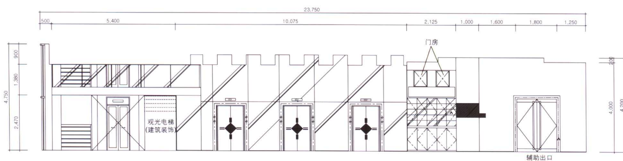
立面图A
