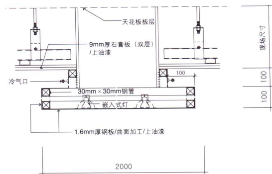
剖面图A
