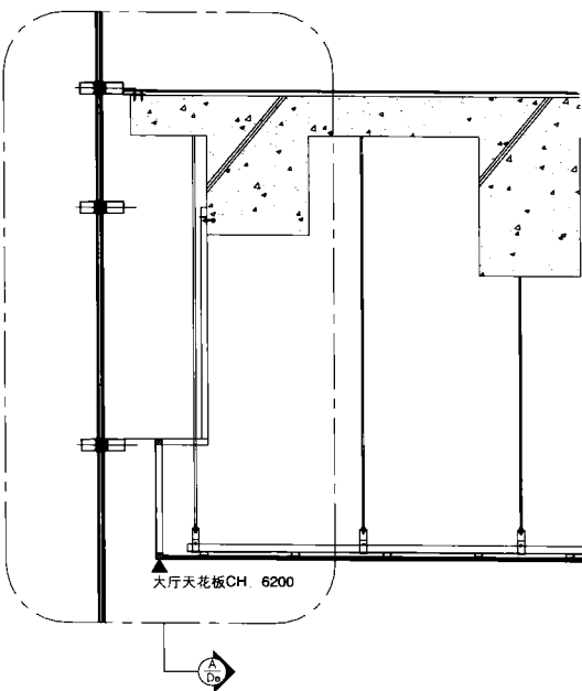
窗帘盒—剖面图
