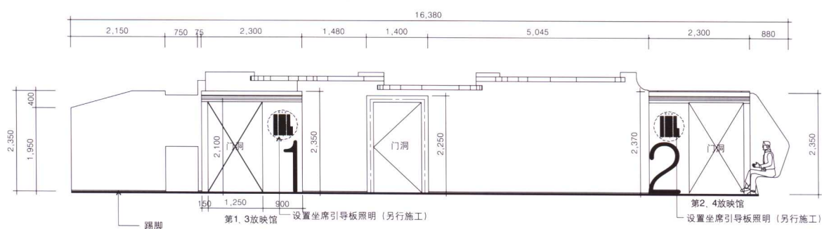
立面图
