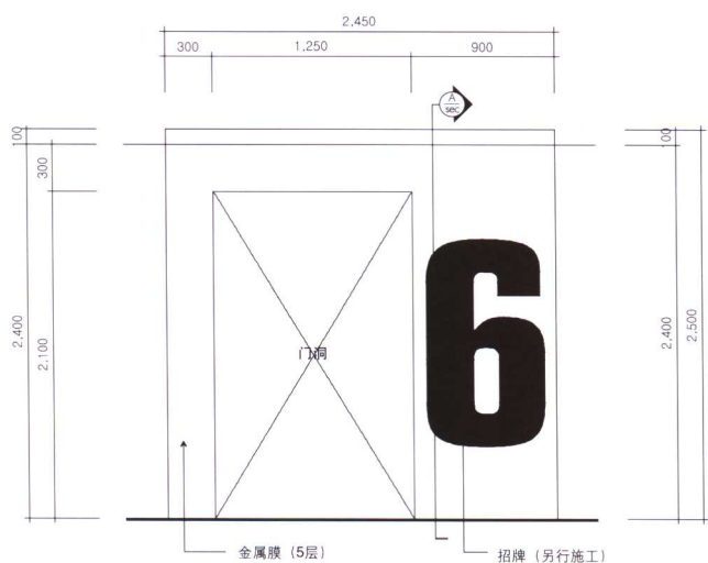
立面图
