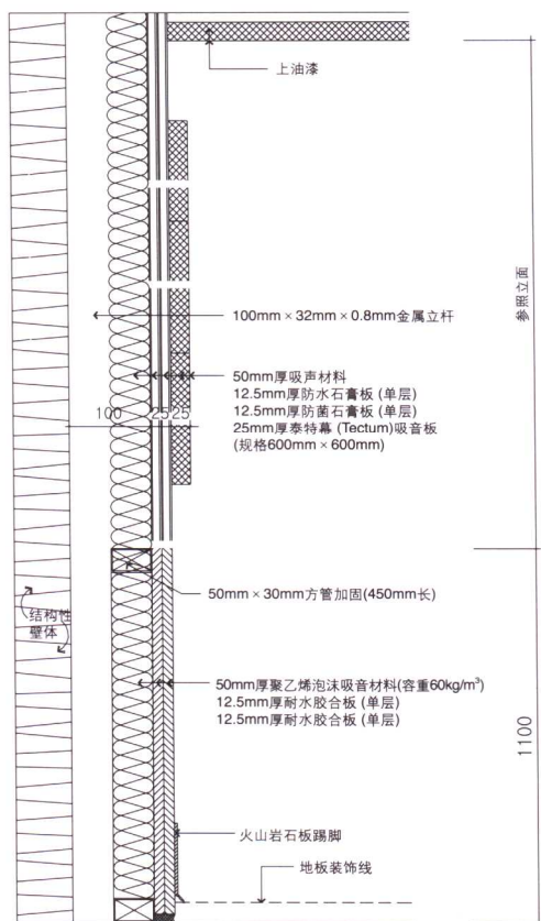
墙体一剖面图
