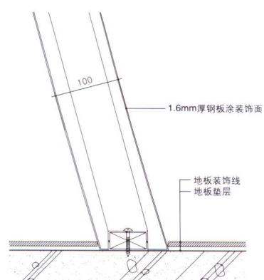
大样图B
