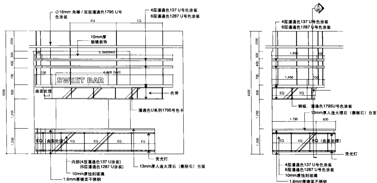
立面图
