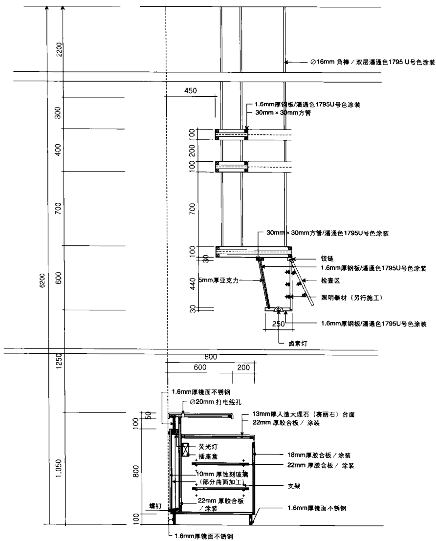
剖面图A
