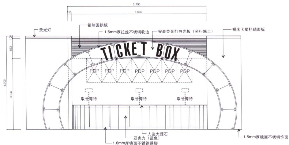
1层售票台-立面图
