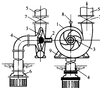
图 1-1 单级单吸式离心泵构造
