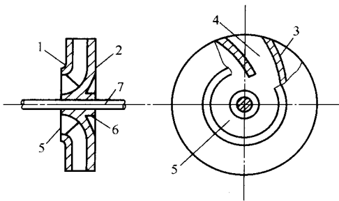
图 1-2 单吸式叶轮
