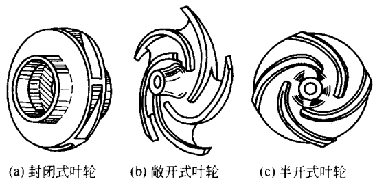
图 1-4 叶轮形式
