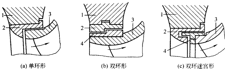
图 1-7 减漏环
