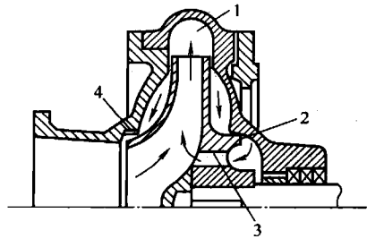
图 1-9 轴向力平衡措施 1—排出压力；2—加装的减漏环； 3—平衡孔；4—泵壳上的减漏环
