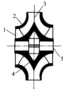
图 1-3 双吸式叶轮
