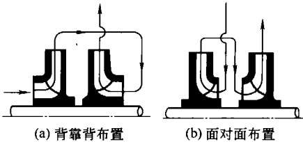
图 1-10 叶轮对称布置
