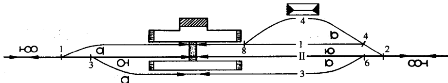
图 1-2 单线铁路中间站布置示意图
