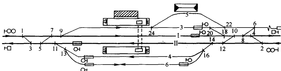
图 1-3 双线铁路中间站布置示意图
