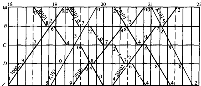
图 1-8 十分格列车运行图(示例)
