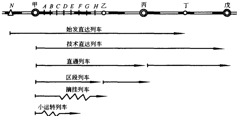
图 1-7 货物列车分类示意图
