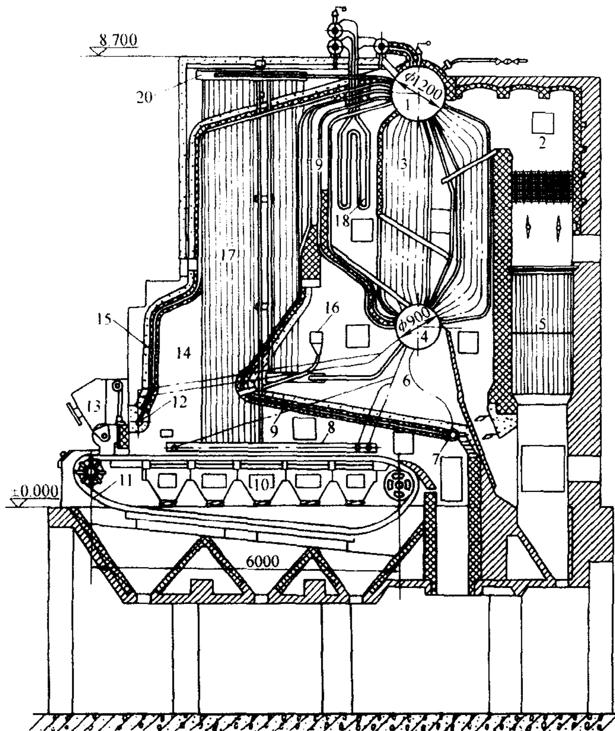
图 1-1 SHL 型锅炉
