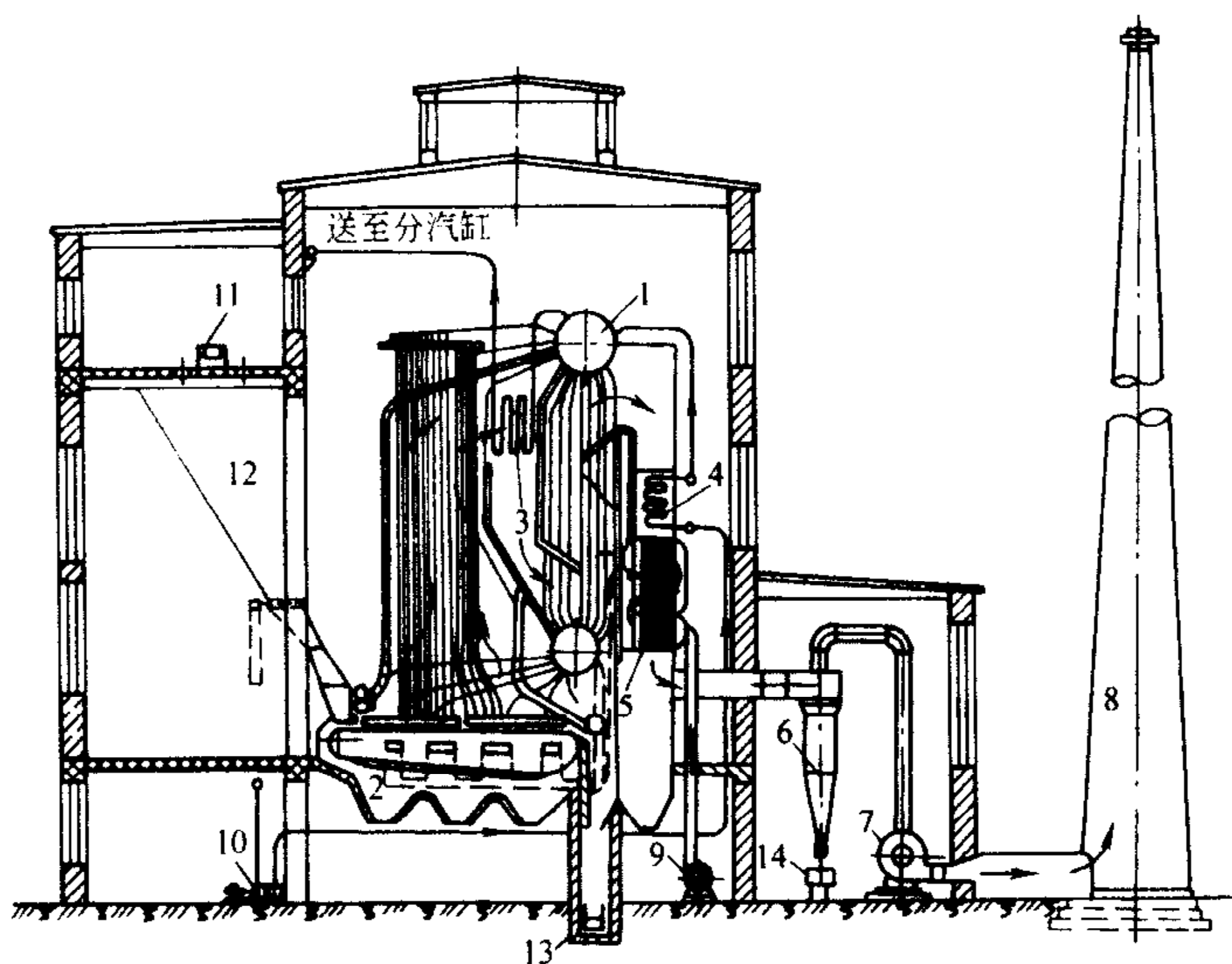
图 1-2 锅炉设备工作过程简图
