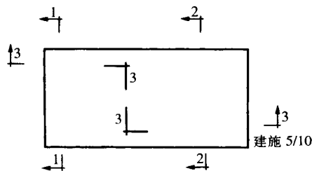
图 1-14 剖切标志方法
