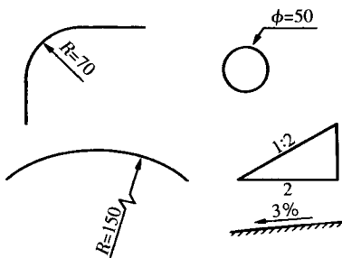
图 1-19 直径坡度标志法
