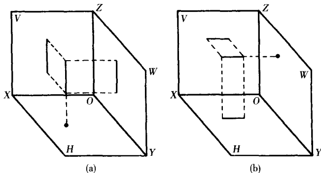
图 1-5 线的投影
