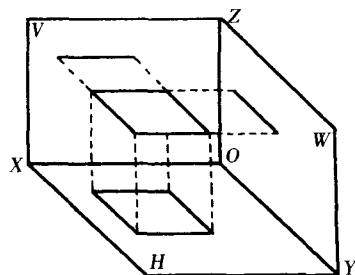
图 1-6 面的投影
