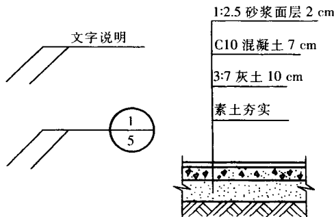
图 1-20 引出线
