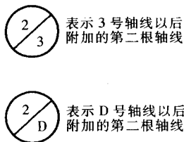
图 1-13 附加轴线标志法
