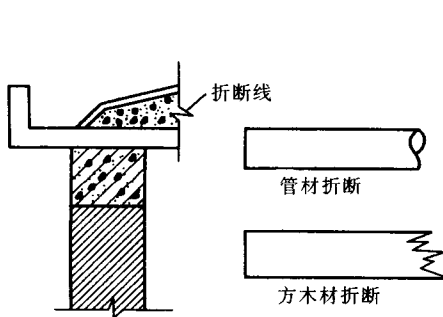
图 1-21 折断线表示方法
