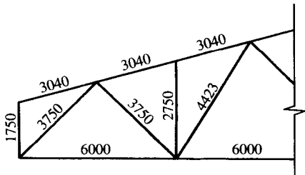
图 1-18 单线图
