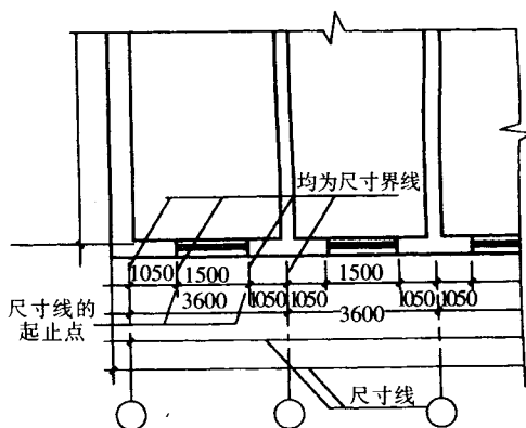
图 1-17 尺寸线标法
