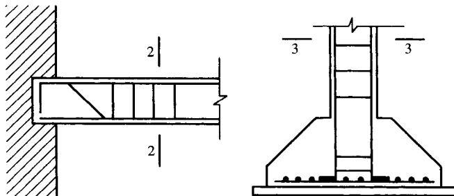
图 1-15 剖视号的标志方法
