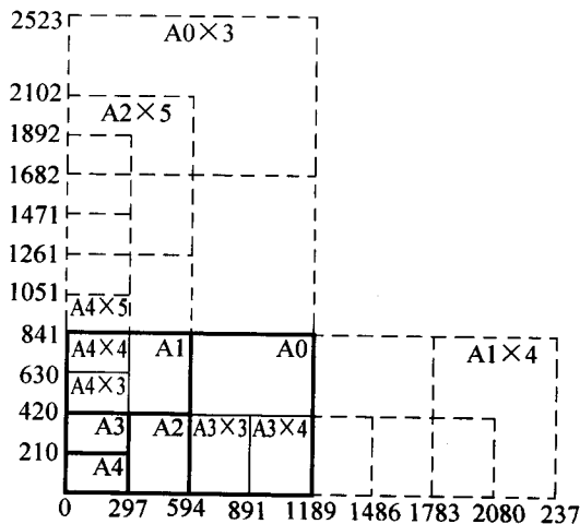
图 1-8 图纸的基本幅面及加长幅面尺寸
