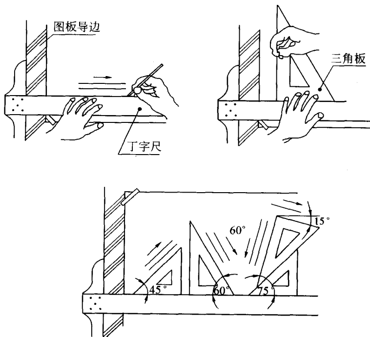
图 1-3 图板、丁字尺和三角板
