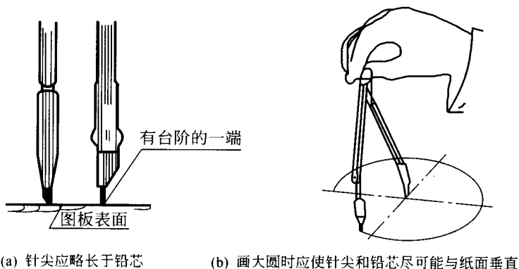
图 1-4 圆规的用法
