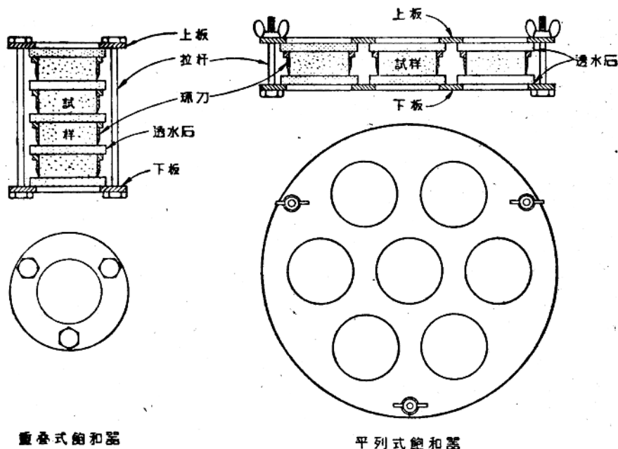
图2 饱和器
