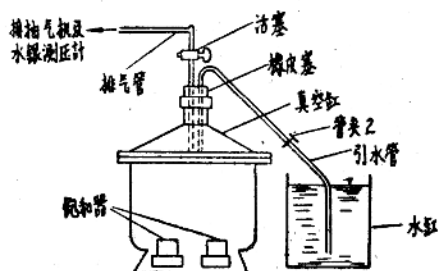
图3 真空饱和法装置
