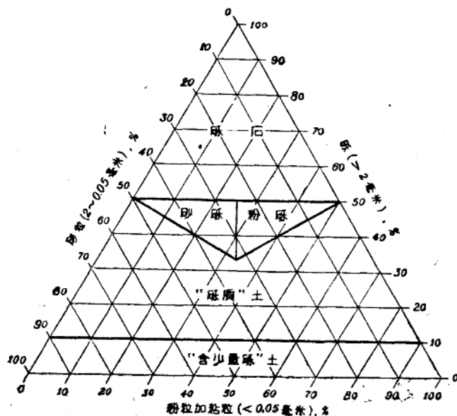
图 2 砾质土分类
