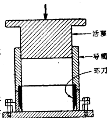
图 1 击实筒
