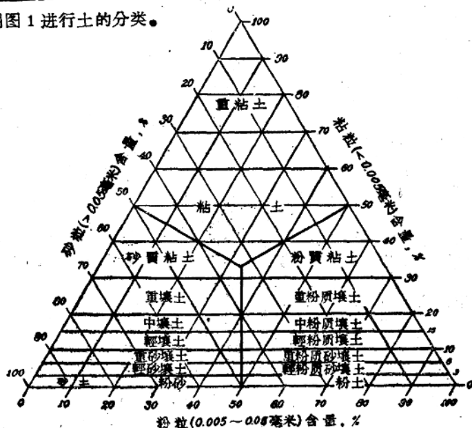
图 1 土的分类
