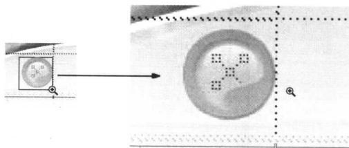
图 1-2 放大页面
