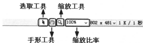
图 1-1 缩放工具
