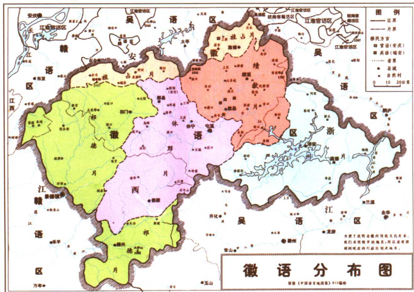
徽语分布图
