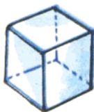
正方体
