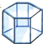
六棱柱体
