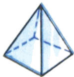
四棱锥体
