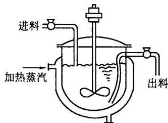
图 1.1 搅拌釜
