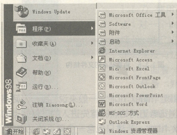
图 1.1.3 启动FrontPage
