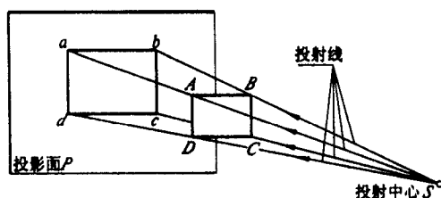
图 1.1 中心投影法
