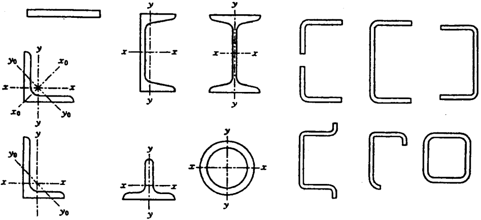
图 1.2.2 轧制和模压型钢
