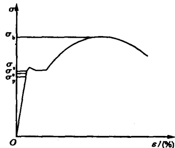
图 1.1.1 钢材的应力—应变图
