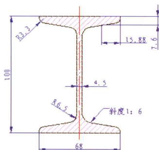
工字钢
