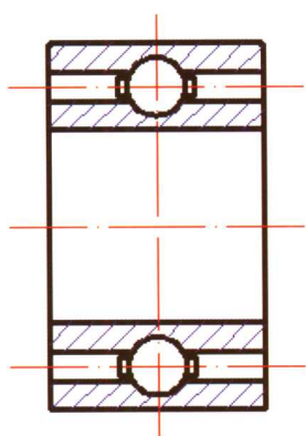
滚动轴承
