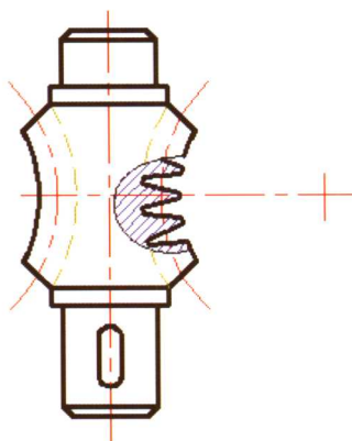
蜗杆
