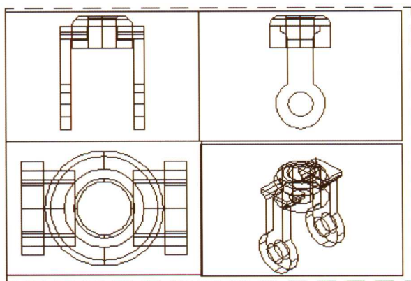
吊架
