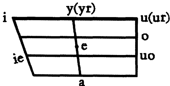
凉山彝语元音舌位图
