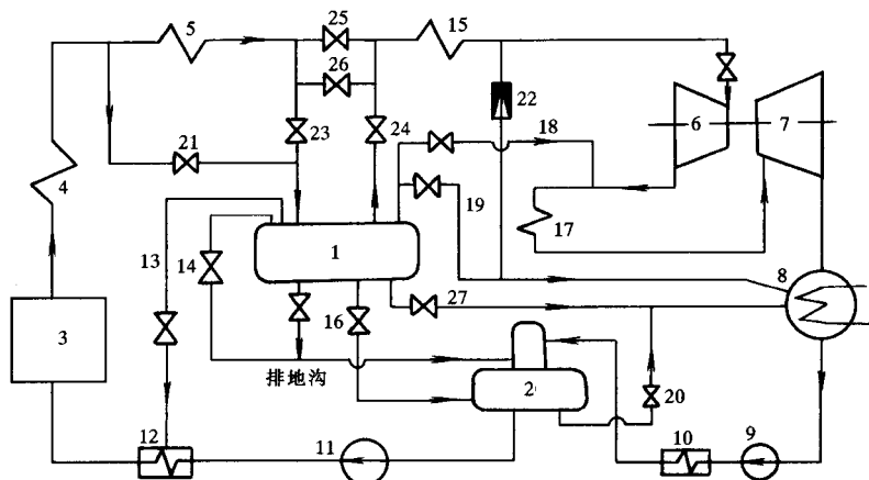
图 1-5 1000t/h 亚临界压力直流锅炉外置式启动旁路系统
