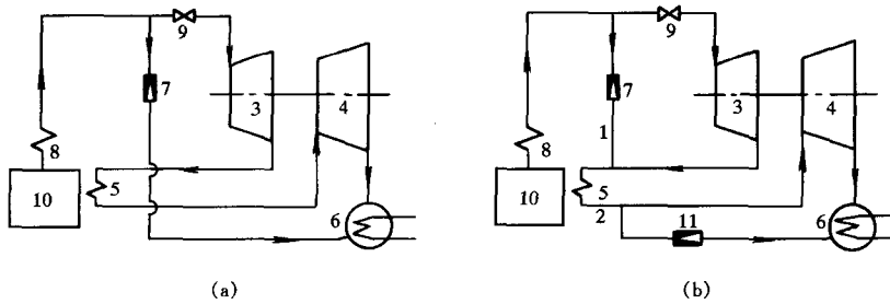
图 1-2 汽轮机旁路系统
