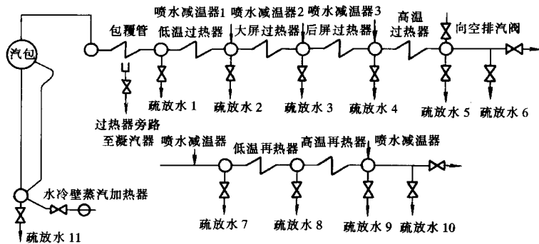
图 1-1 自然循环汽包锅炉典型汽水系统与疏放水系统
