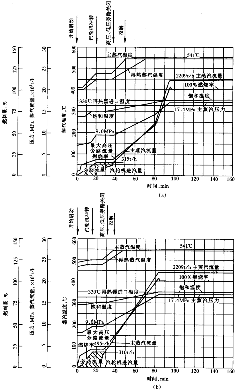
图 1-4 德国 BABCOCK-2208t/h 自然循环锅炉热态和极热态启动曲线 (a) 热态启动；(b) 极热态启动
