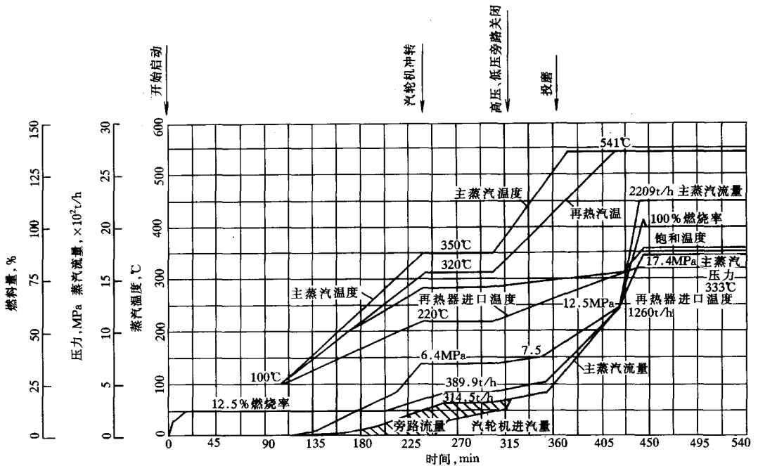
图 1-3 德国 BABCOCK-2208t/h 自然循环锅炉冷态滑参数启动曲线
