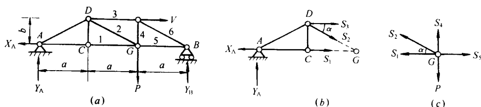
图 5-7 截面法解桁架受力
